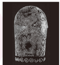
太刀の柄頭(X線CT写真)
